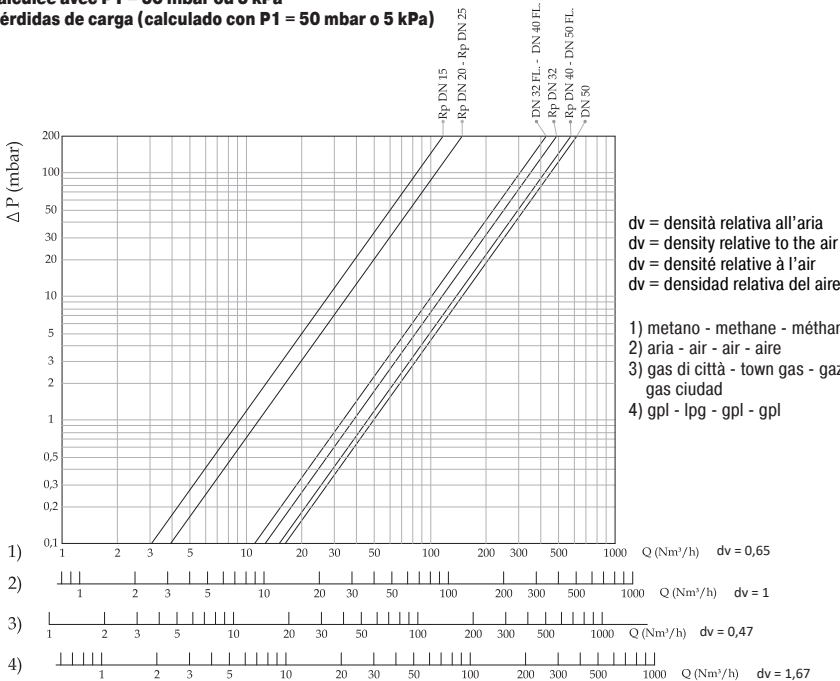
Diagramma calcolato con P1 = 50 mbar o 5 kPa Pressure loss diagram (calculated with P1 = 50 mbar or 5 kPa) Schéma calculée avec P1 = 50 mbar ou 5 kPa Tabla de pérdidas de carga (calculado con P1 = 50 mbar o 5 kPa)
