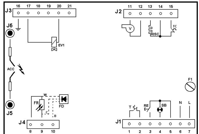
Type TGRD71
